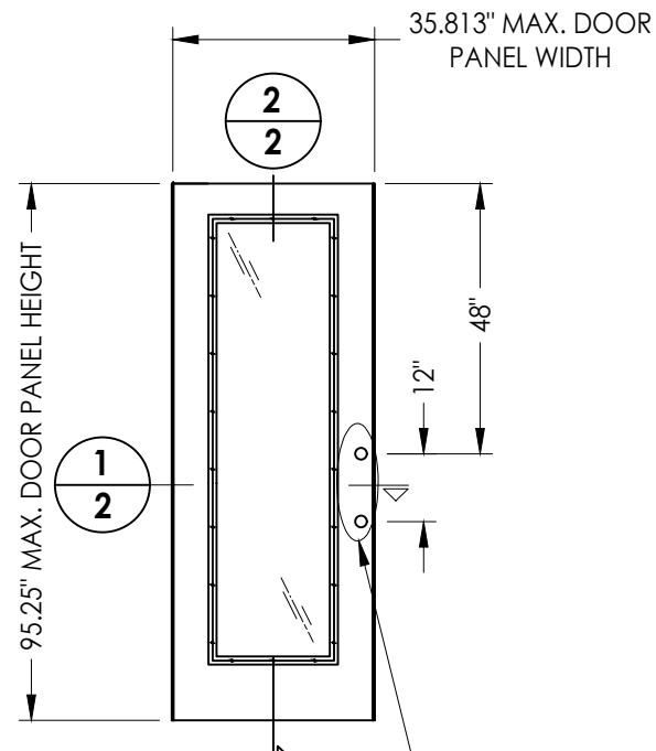
41 DOOR PANEL Hybrid Door
